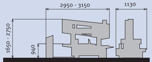
Dimensions BMBS 460 x 600 HA-DG-F
