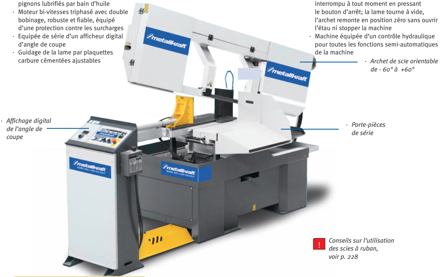
Fig.: BMBS 460 x 600 HA-DG-F
