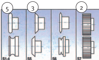
S1-4: molettes standard pour Ø 3/6/8/10 mm
